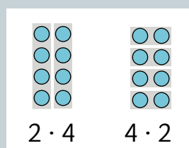
2 \times 4 und 4 \times 2 mit den Punktestreifen
