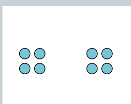
2 \times 4 als Punktemuster
